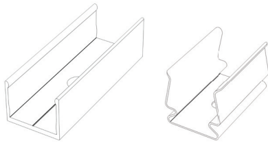
Clip 50 mm
