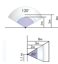
Indoor 140-L
