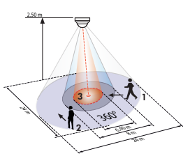
PD4N-1C
