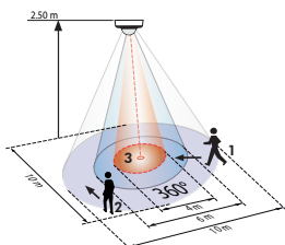
PD3, PD3N
