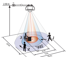
PICO-tunnistin
