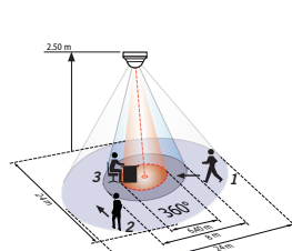
PD4-tunnistimet
