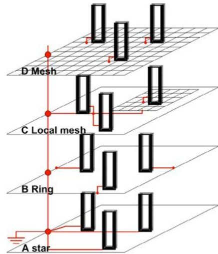
EN 50310 Minimum
