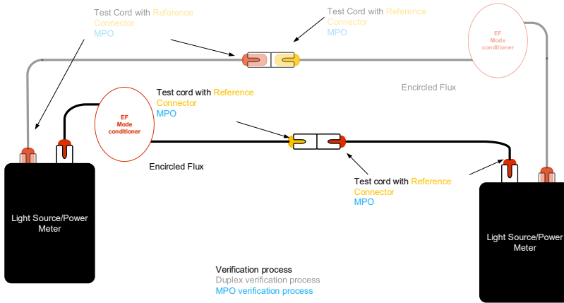
«one Jumper» method verification
