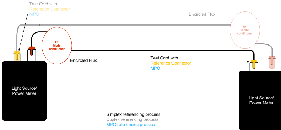
«one Jumper» reference method
